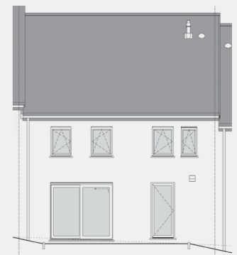
Façade arrière
